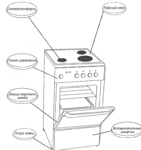
Трехконфорочная электроплита Рис. 1. Общий вид электроплиты
