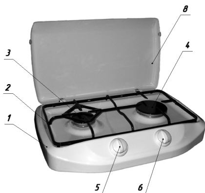
Рис. 1 Устройство плиты
