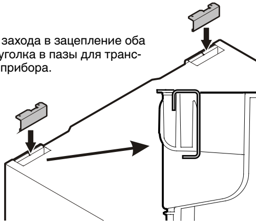
Вид сбоку
