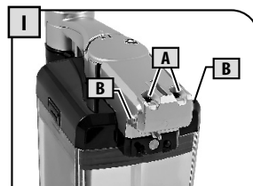
A = Отверстия графина B = Штыри графина
