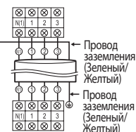
Внутренний блок
