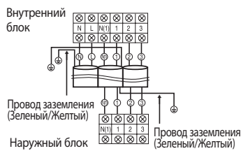
Наружный блок
