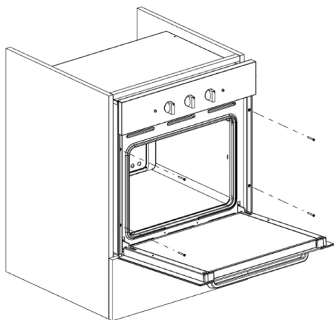
Рис. 7. Схема по встраиванию духового шкафа
