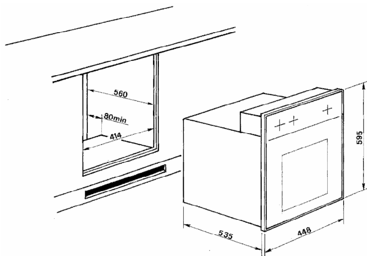
Рис. 7. Схема по встраиванию духового шкафа
