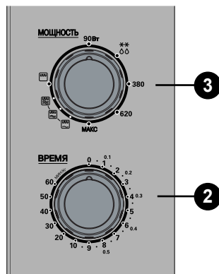
MH-6327DR MH-6327DRS
