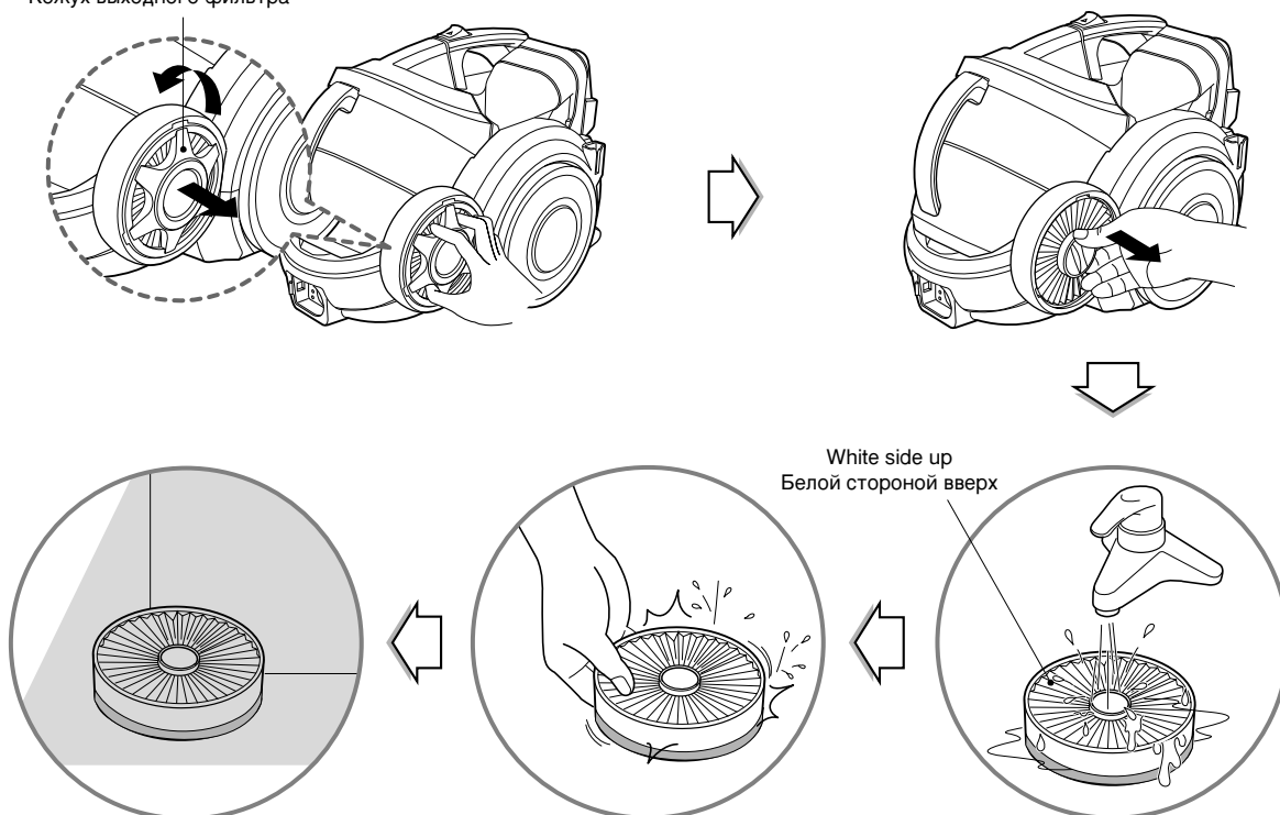
Exhaust filter cover Кожух выходного фильтра
