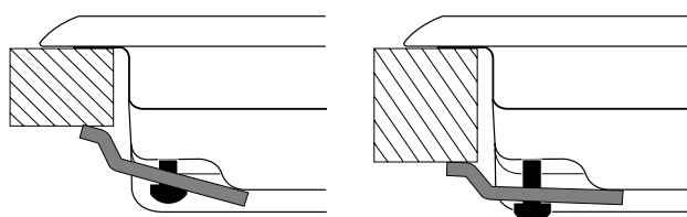
прилагающиеся крюки. Схема крепления крюков
