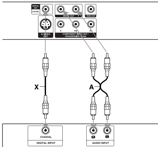
Усилитель (ресивер)
