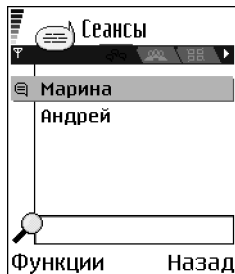
Рис. 16 Экран "Сеансы"
