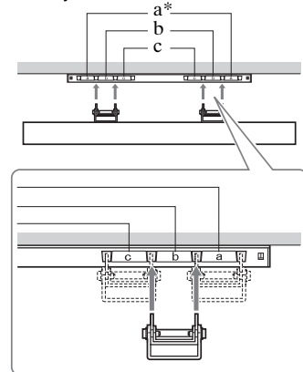
Розташування гаків
