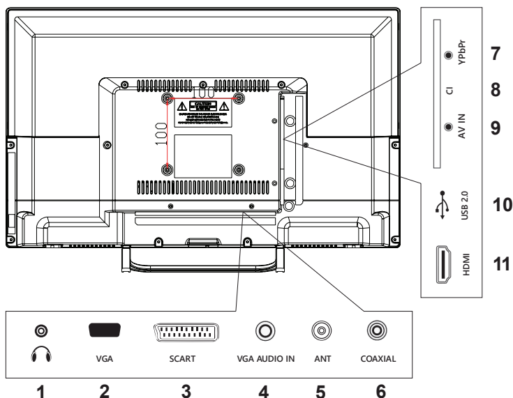
Рисунок 4 – ВИД ТЕЛЕВИЗОРА СЗАДИ, НАЗНАЧЕНИЕ РАЗЪЕМОВ ДЛЯ ВНЕШНИХ ПОДКЛЮЧЕНИЙ
