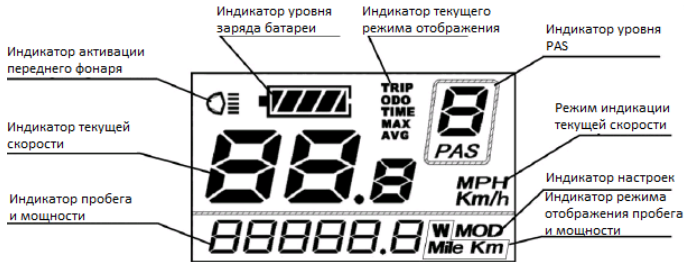
Рисунок 8. Структура дисплея LCD-пульта
