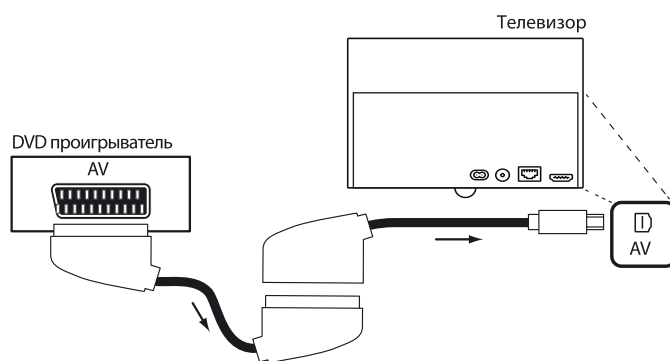
Пример подключения DVD проигрывателя
