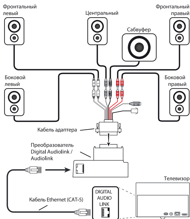
Подключение активной акустической системы к телевизору
