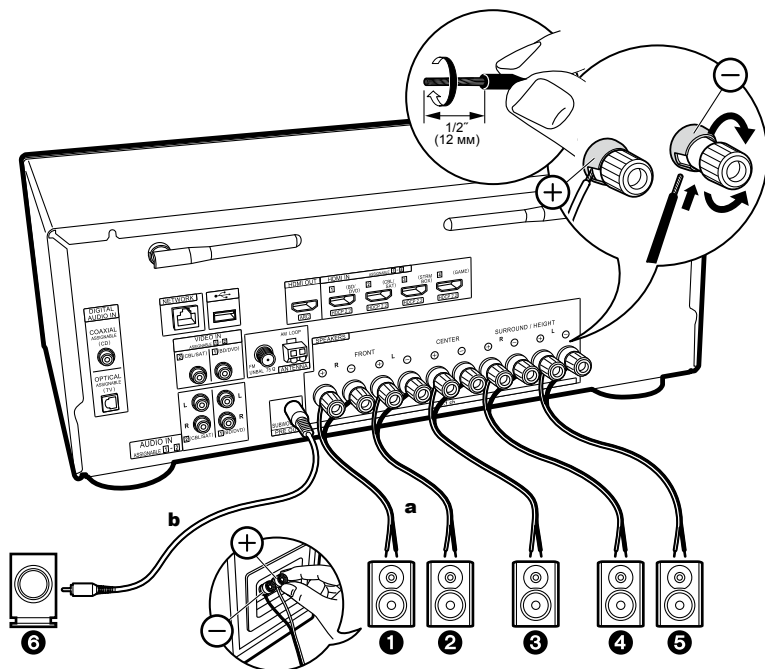
a Кабель подключения АС, b Кабель сабвуфера
