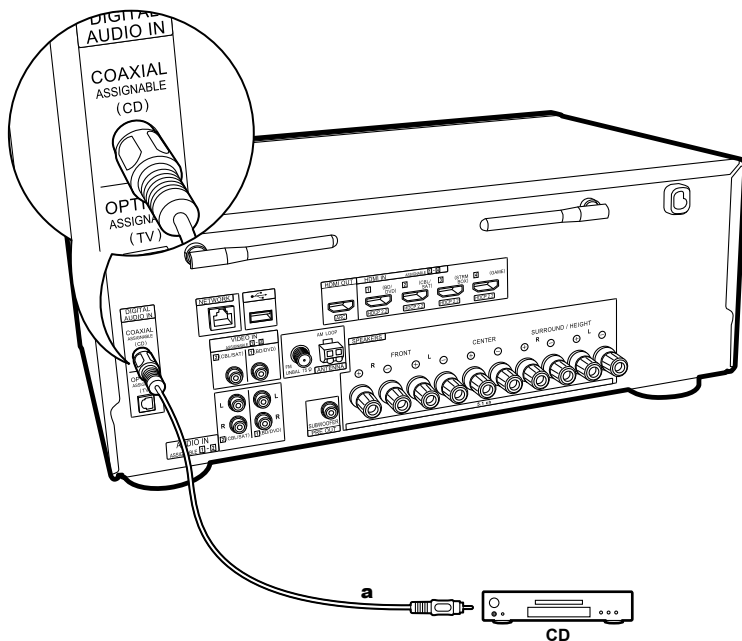
a Цифровой коаксиальный кабель
