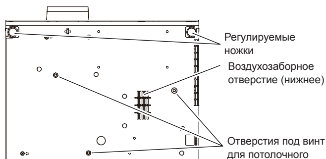
Места расположения регулируемых ножек и отверстий под винты для потолочного крепления
