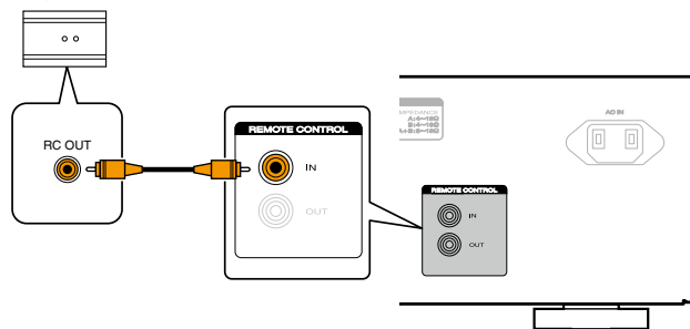
ИК-приемник
