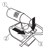
① Mikrofon ② Mikrofonklemme ③ Mikrofonsockel
