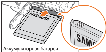
Аккумуляторная батарея
