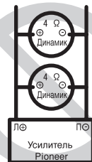
Мостовое соединение 2 Ω
