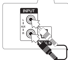
Задняя панель устройства
