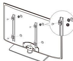
В жағдайы. Басқа компания шығарған қабырғалық аспа жинақты орнату
