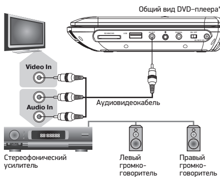
Рис.5. Подключение к стереофоническому усилителю
