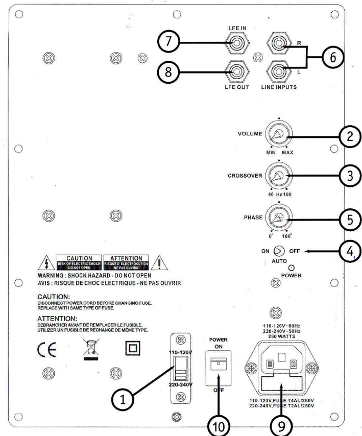
2011 + Вид сабвуфера серии Impression.
