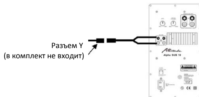
Рисунок 2. Подключение к выходу Subwoofer или LFE аудио/видео ресивера или усилителя.
