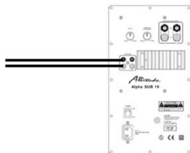
Рисунок 3. Подключение к левому и правому выходам Line Level от A/V ресивера или усилителя.
