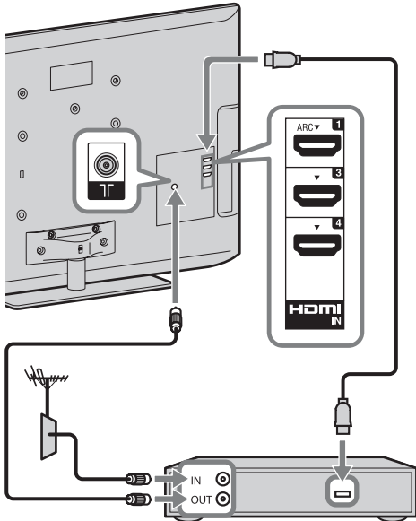
ТВ-ресівер/записуючий пристрій (наприклад, DVD-рекордер)
