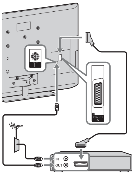
Телеприставка/видеозаписывающее устройство (например, DVD-рекордер)
