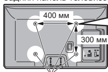
Отверстия для крепления настенного кронштейна
