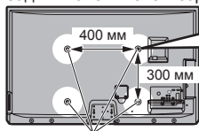
Отверстия для крепления настенного кронштейна
