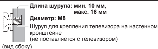
Отверстия для крепления настенного кронштейна
