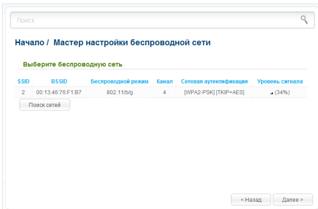
Рисунок 76. Страница выбора сети для подключения.
