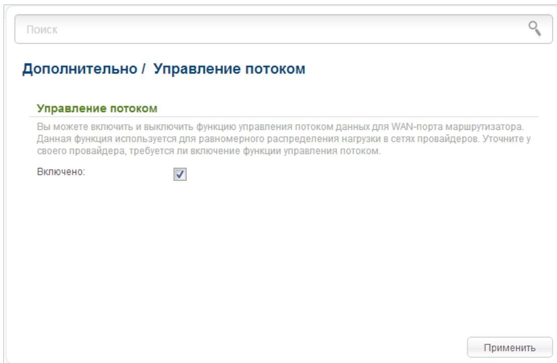
Рисунок 145. Страница Дополнительно / Управление потоком .
