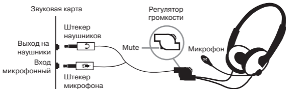
Рис. 1. Схема подключения
