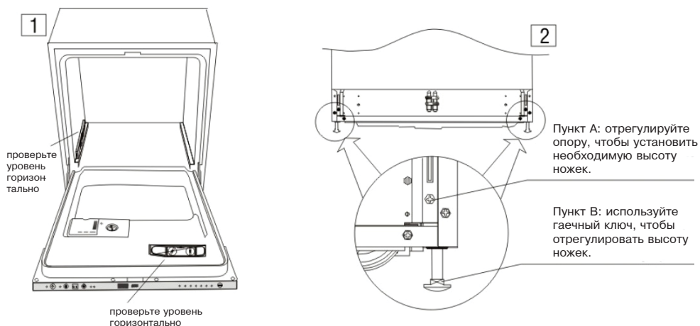
Рис. 8. Регулирование горизонтального положения машины
