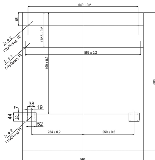
Рис. 3. Для модели BDE 6007. Все размеры приведены в мм.
