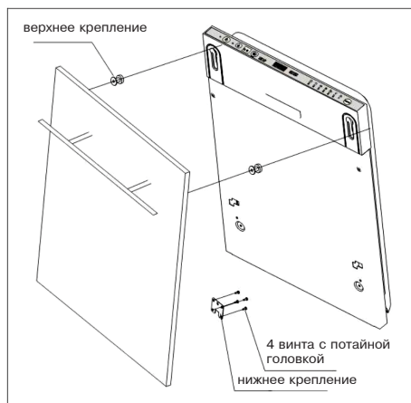
Рис. 4а. Установка декоративной панели.
