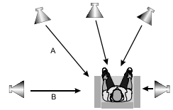
Рис. 1. Учитывайте расстояние между A и B, используйте оба рисунка для правильного расчета значения задержки.
