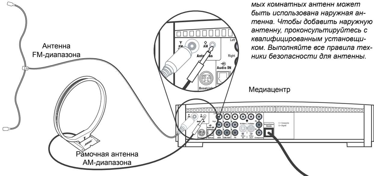
Рисунок 10 Подсоединения антенн
