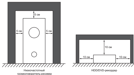
Низкочастотный громкоговоритель-ресивер
