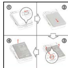
Извлечение батареи
