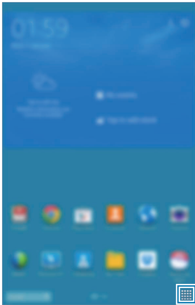
<Главный экран>
