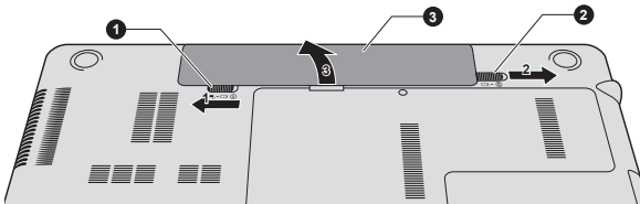
Рисунок 5-1 Высвобождение батарейного источника питания – 1
