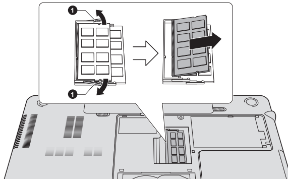
Рисунок 3-15 Удаление модуля памяти
