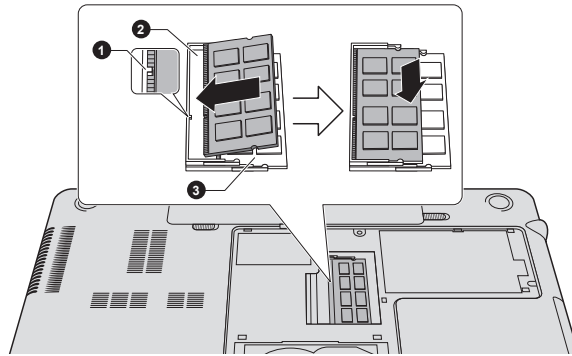
Рисунок 3-13 Установка модуля памяти
