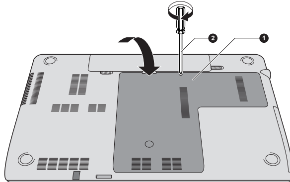
Рисунок 3-14 Установка крышки отсека модулей памяти
