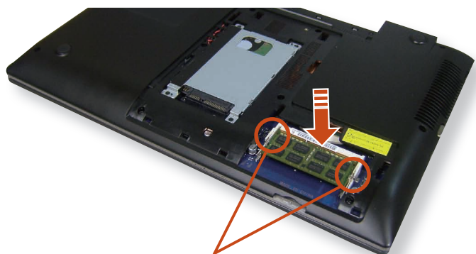
Защелки модуля памяти
