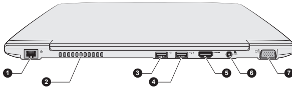
Рисунок 2-4 Вид компьютера сзади
