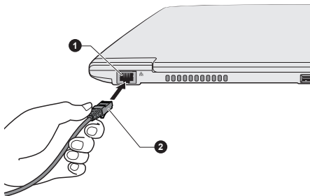
Рисунок 3-6 Подключение сетевого кабеля
