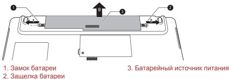
Рисунок 5-1 Высвобождение батарейного источника питания (L770/L775/L770D/L775D)
