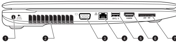
Рисунок 2-8 Левая сторона компьютера
