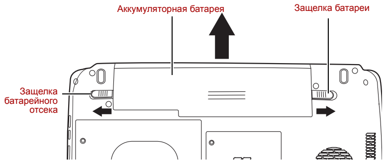
Высвобождение батарейного источника питания
