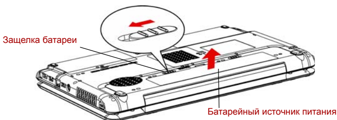
Рисунок 6-2 Снятие батарейного источника питания
