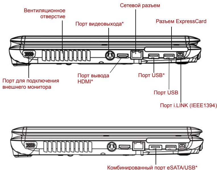
Рисунок 2-2 Вид компьютера слева
