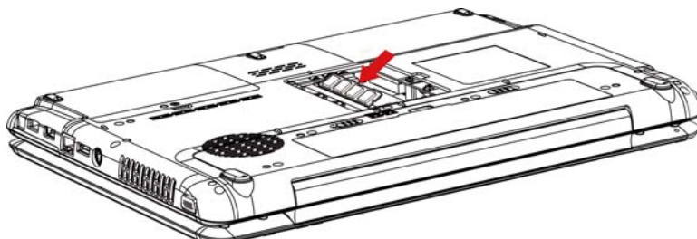
Рисунок 8-8 Установка модуля памяти в разъем
