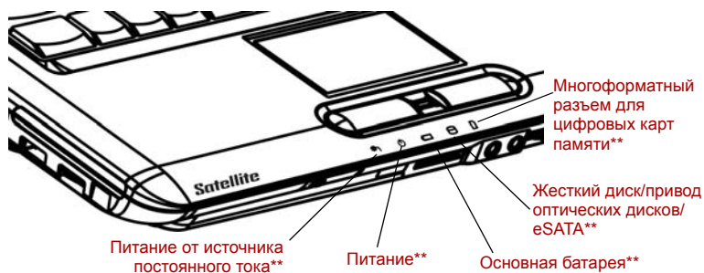
Рисунок 2-7 Системные индикаторы
