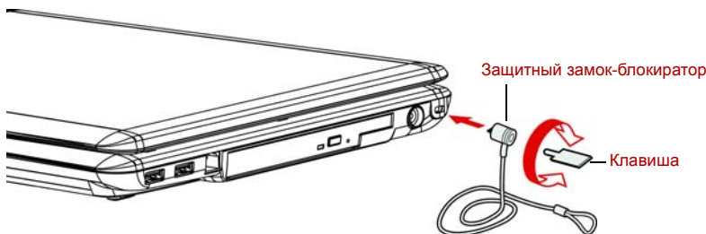
Рисунок 8-13 Защитный замок-блокиратор
