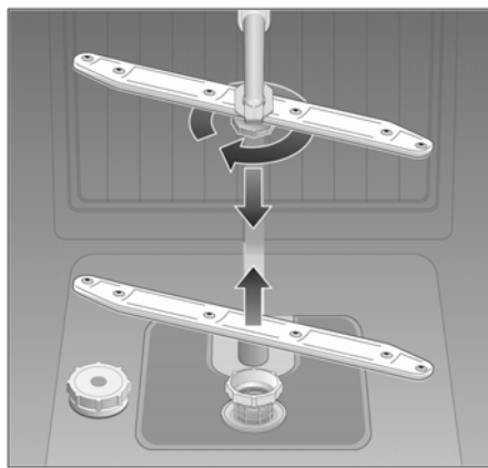
Распылительные коромысла
