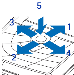
Рис. 2 Клавиша прокрутки
