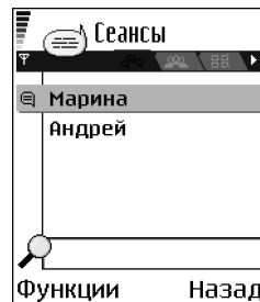
Рис. 19 Экран "Сеансы"
