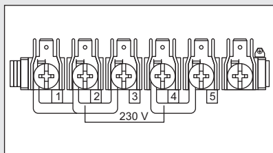
Клеммная колодка
