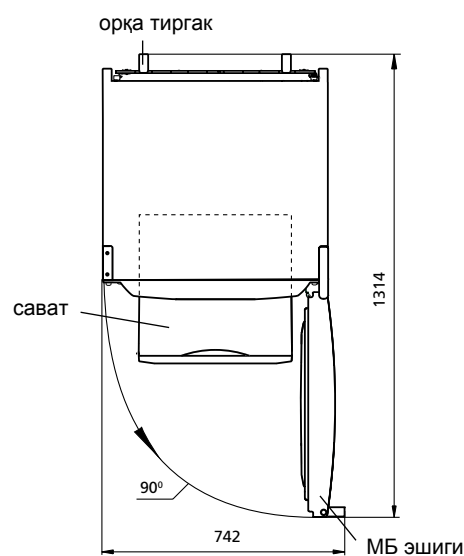
2-расм — Совутқич (уст қисми) кўриниши
