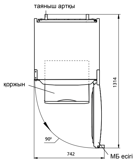
2 сурет — Тоңазытқыш (жоғарыдан көрініс)
