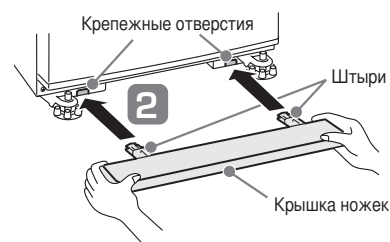
Крепежные отверстия
