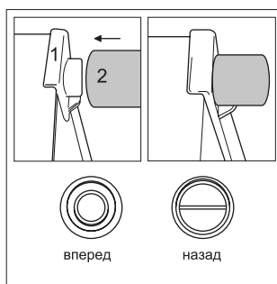
Рис. 1. Установка ограничительных упоров
