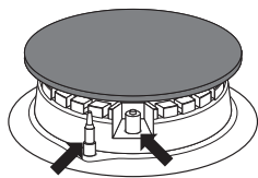
Датчик пламени*
